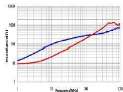
CMZ4520A-901&102T
