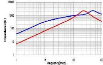
CMZ4520A-901&102T
