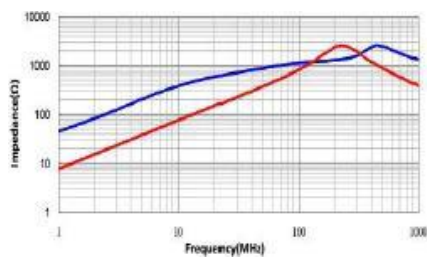
CMZ4520A-122T
