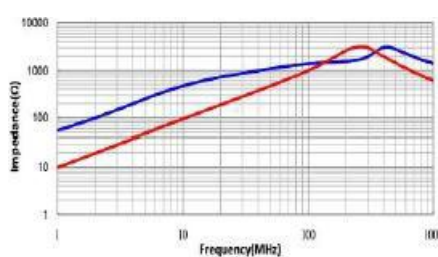
CMZ4520A-142T
