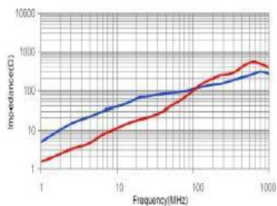
CMZ4520A-401&421T
